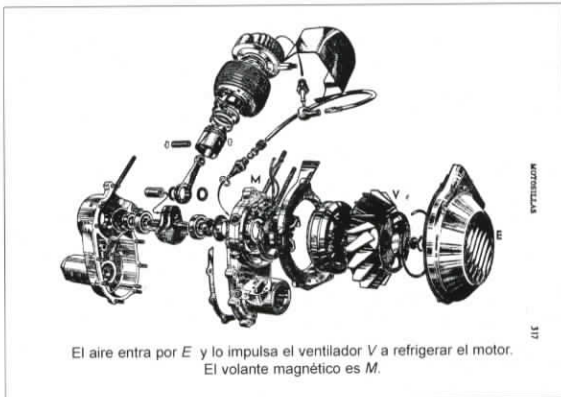
Motor de la Vespa despiezado
