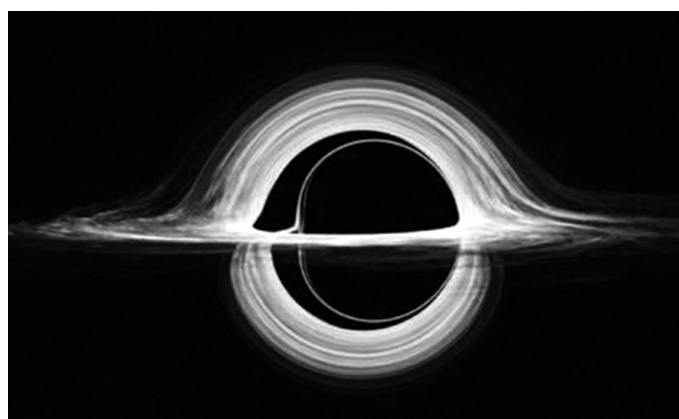
INTERSTELLAR. Imagen distorsionada de un agujero negro rotante y con disco de acreción.
